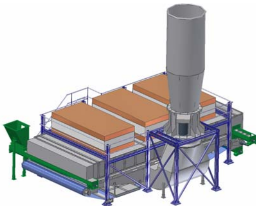
Abbildung 4 3-D Zeichnung KUV0 mit 2-stufiger Warmluftferzeugung
